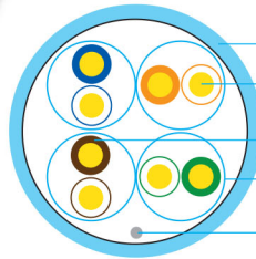
US-9256LSZH U/FTP
