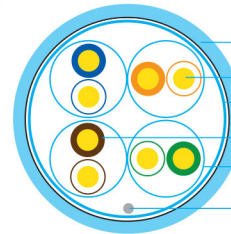
US-9267LSZH F/FTP
