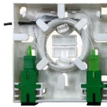
LINK F.O. Mini FTTH Outlet (for 2xSC Simplex or 2xLC Duplex)
